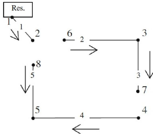
Слика 3. Схема мреже са уклоњеним изолационим затварачима; стрелицама су обележени претпостављени смерови течења у цевима
