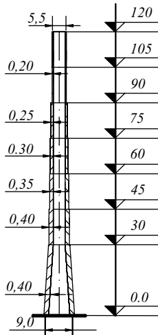
Slika 1. Geometrija dimnjaka
