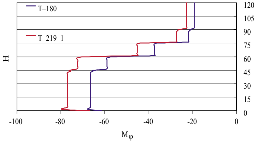
Slika 9. Radijalni momenti savijanjau u dimnjaku pri režimu temperature T-180 i T-219-1
