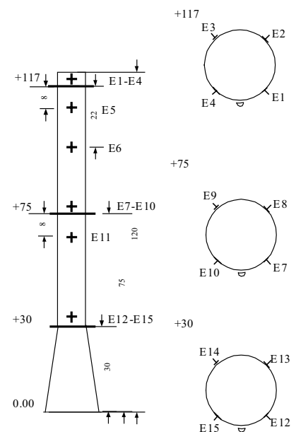
Slika 14. Dispozicija mesta snimanja termoizolacije pomoću video-endoskopa
