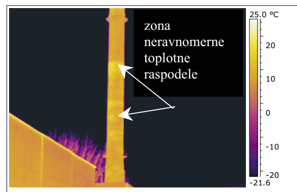
Slika 2. Termografski snimak dimnjaka, [1]
