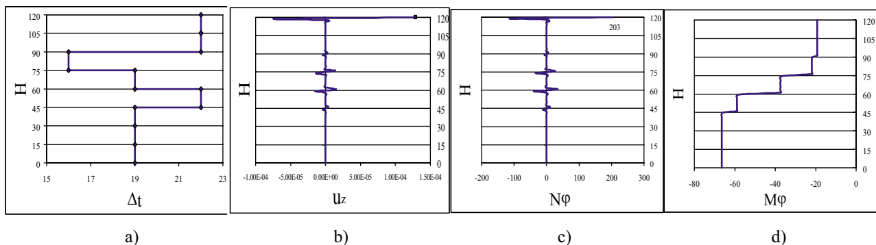
Slika 8. Uticaji u dimnjaku usled \Delta t pri režimu temperature T-180: b) radijalno pomeranje, c) aksijalne sile u radijalnom pravcu, d) radijalni momenti savijanja
