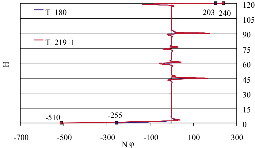
Slika 10. Radijalne sile u dimnjaku pri režimu temperature T-180 i T-219-1
