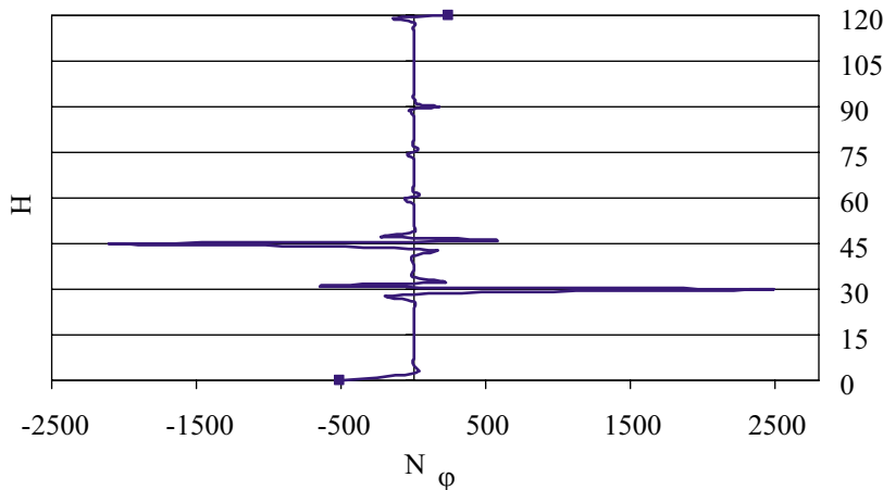
Slika 12. Radijalne sile u dimnjaku pri režimu temperature T-219-2
