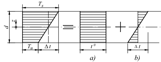
Slika 6. Raspodela temperature po debljini zida ljske
