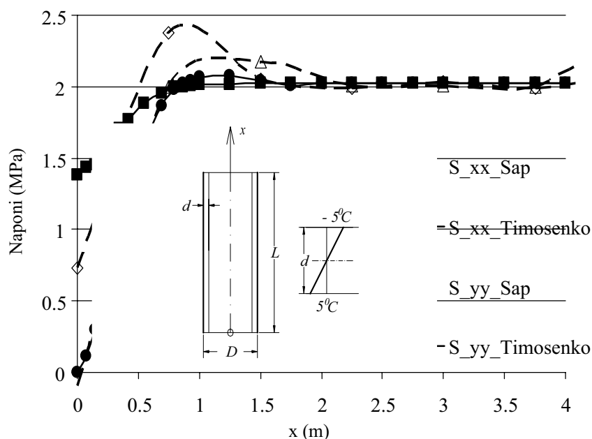
Slika 5. Model dimnjaka
