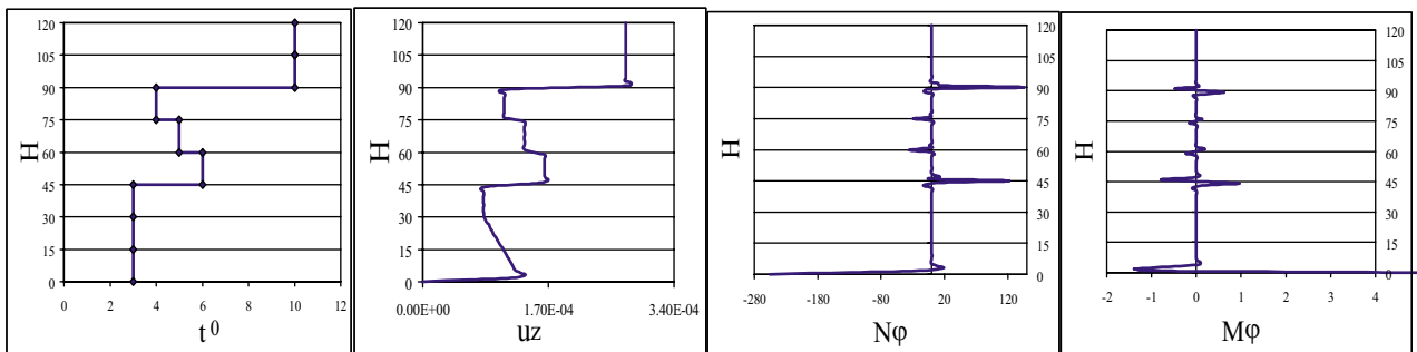
Slika 7. Uticaji u dimnjaku usled t^0 pri režimu temperature T-180: b) radijalno pomeranje, c) aksijalne sile u radijalnom pravcu, d) radijalni momenti savijanja
