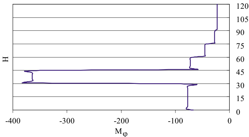
Slika 11. Radijalni momenti savijanjau u dimnjaku pri režimu temperature T-219-2
