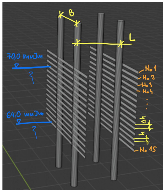
Slika 1. Model dela građevine sa odbojnicima pričvršćenim za šipove Figure 1. Model of the part of the breakwater structure
