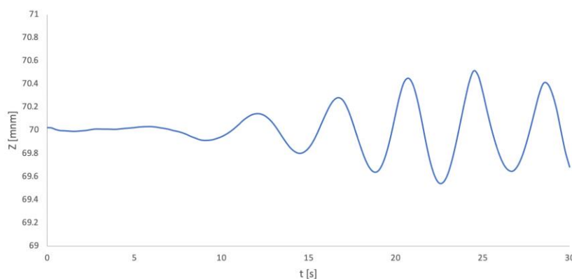
Slika 5. Izlazni nivogram za varijantu sa odbojnicima visine 50 cm Figure 5. Output hydrograph for the variant with the steel plate height of 50 cm
