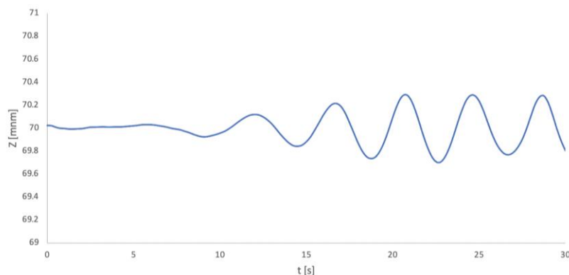
Slika 4. Izlazni nivogram za varijantu sa odbojnicima visine 25 cm Figure 4. Output hydrograph for the variant with the steel plate height of 25 cm
