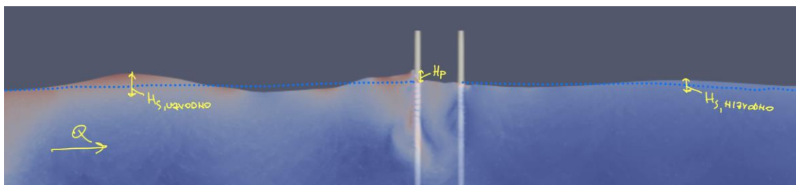
Slika 2. Podužni presek kroz deo računskog domena sa građevinom sa odbojnicima Figure 2. Longitudinal profile of the numerical domain with the breakwater structure Opis SPH metode
