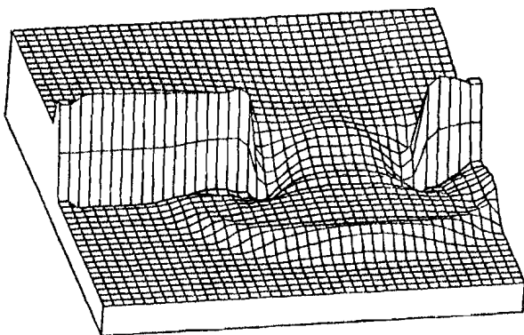
S1. 1. – Ravansko tečenje kao posledica delimičnog rušenja brane ( t=15 s)
