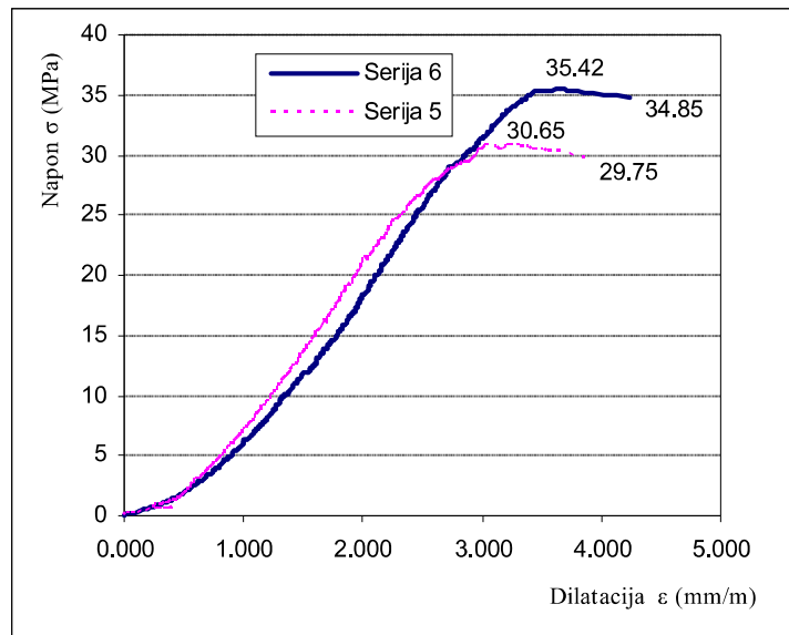
Слика 2. Упоредни приказ \sigma - \varepsilon дијаграма бетона серија "5" и "6"
