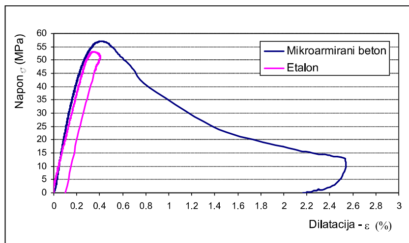
Слика 3. \sigma - \epsilon дијаграми две серије бетона (еталона и микроармираног бетона)
