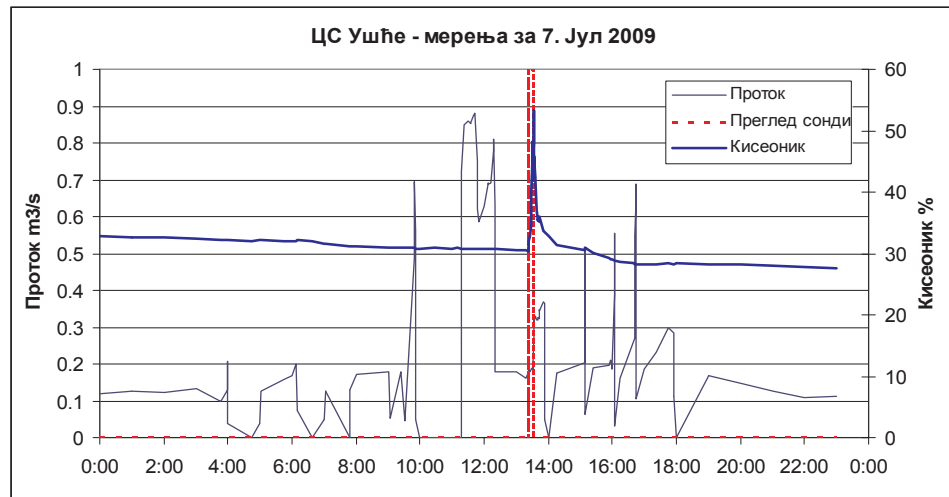
Slika 7. U SCADA-i postoji i informacija o trenutku kalibracije sonde Figure 7 SCADA gives information about the moment of plug calibration
