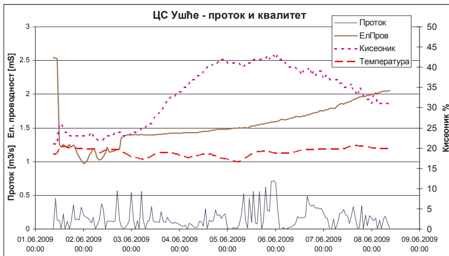
Slika 6. Rezultati merenja kiseonika, temperature vode i elektroprovodnosti na CS Ušće, od 1.-9. juna 2009.
