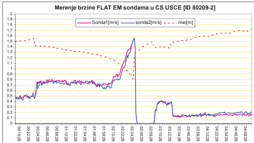
Slika 3. Brzine u tunelu ispred CS Ušće (9. februar 2009) – sirov signal sa dve sonde za brzinu i nivo \Delta t=1\text{min}
