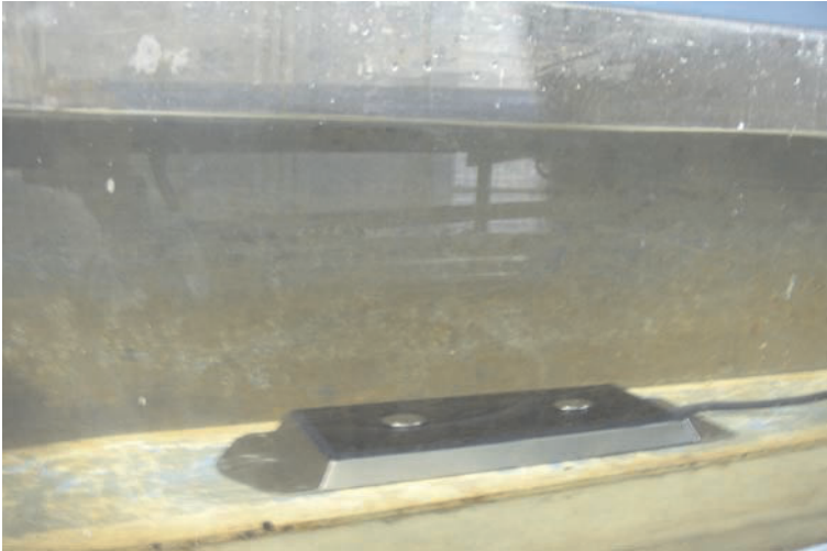
Slika 1. Ravna EM sonda tokom ispitivanja u laboratorijskom kanalu Figure 1 Flat EM plug during the examinations in laboratory channel
