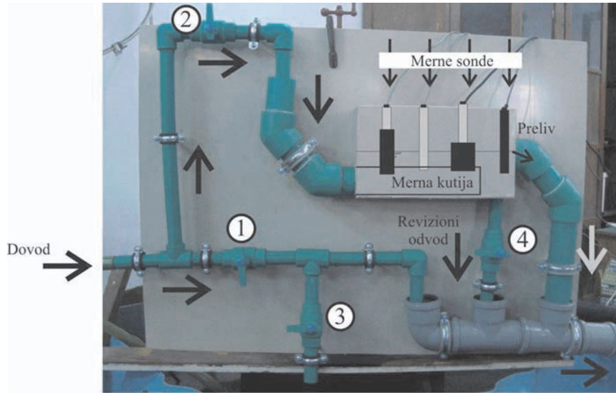
Slika 5. Kutija za smeštaj sondi za kvalitet sa sistemom za dovođenje i odvođenje vode
