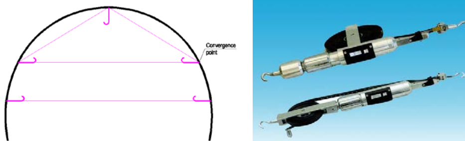
Слика 9. Мјерење радијалних деформација мјерењем дужина
