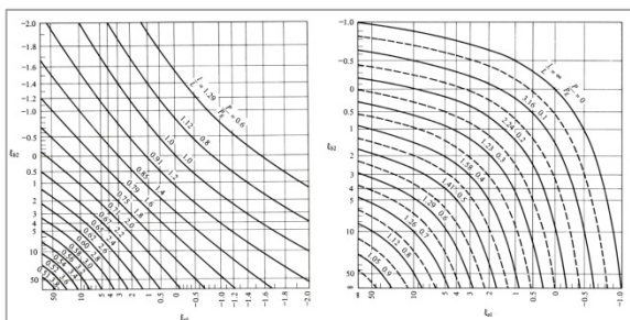
Слика 3. Критично оптерећење еластично ослоњеног штапа са непомерљивим и померљивим чворовима [1]
