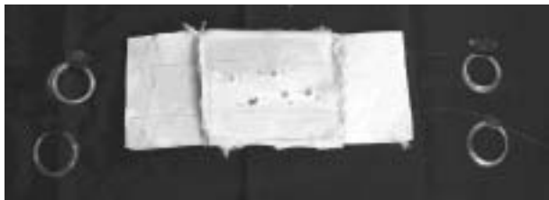
Slika 2. Fotografija kompozitne ploče sa ugrađenim optičkim vlaknima nakon pet balističkih testiranja
