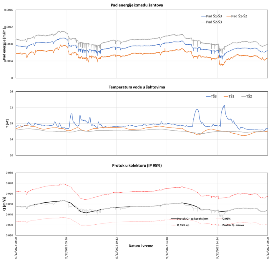
Slika 5. Stara Pazova: Gore) Promena pada energije između šahtova; Sredina) Promena temperature vode u šahtovima; Dole) Promena protoka u kolektoru sa intervalom poverenja od 95%
