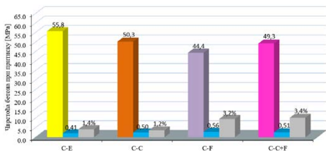
Сл. 6. Чврстоће бетона при притиску у старости од 28 дана са приказом вриједности водоцементног фактора и процента увученог ваздуха
