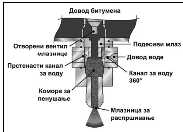
Слика 9. Шема млазнице за пенести битумен [2]
